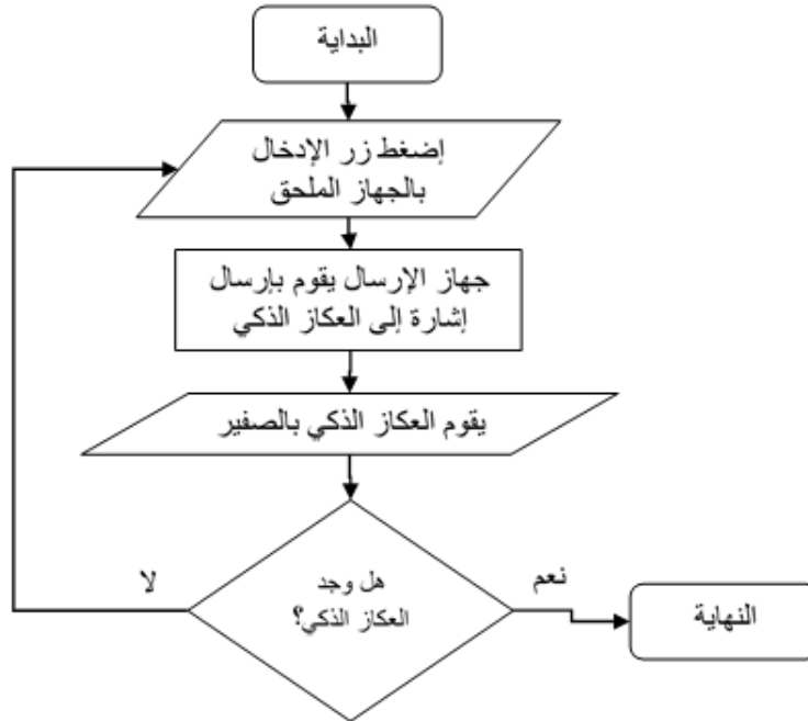
الشكل 2. المخطط الانسيابي لنشاط جهاز التنبيه الملحق بالعكاز الذكي
