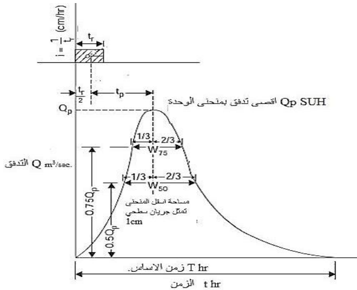
شكل (1) خصائص منحنى الوحدة للتدفق (Synthetic Unit Hydrograph) حسب نموذج سنيدر Snyder's Model [7].
