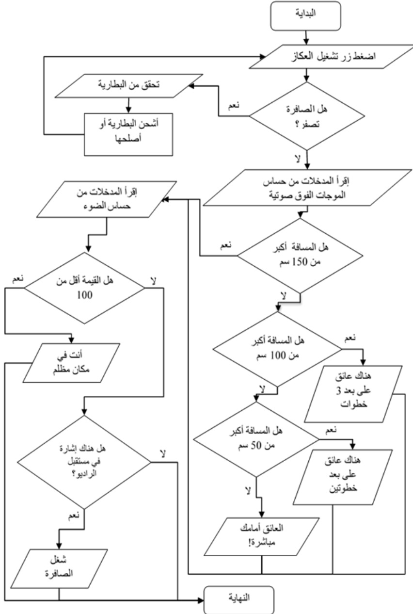
الشكل 3. المخطط الانسيابي لدورة واحدة لنشاط جهاز العكاز الذكي
