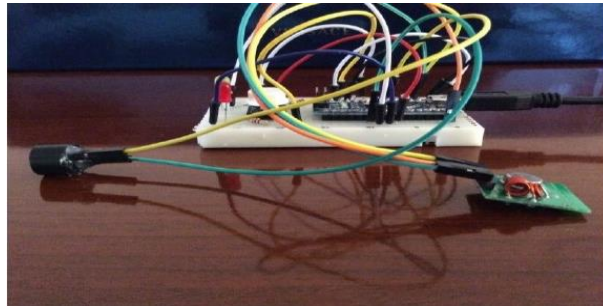
الشكل 5. لوحة جهاز التنبيه الملحق بالعكاز الذكي بعد تجميعها.
