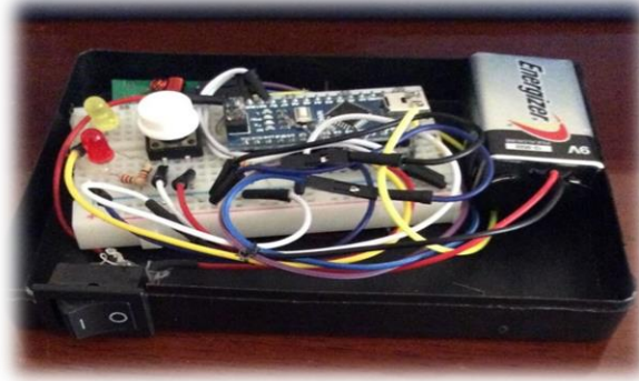
الشكل 4. لوحة جهاز العكاز الذكي بعد تجميعها.
