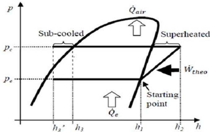
p-h diagram شكل (2) يوضح دورة التبريد للتلاجة المصدر : مرجع رقم [3]
